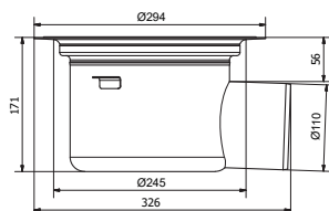
Sida Ø110 mm (Syrafast rostfritt stål)
