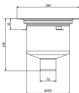
Botten Ø75 mm (Syrafast rostfritt stål)
