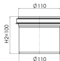
Botten Ø110 mm (Syrafast rostfritt stål)
