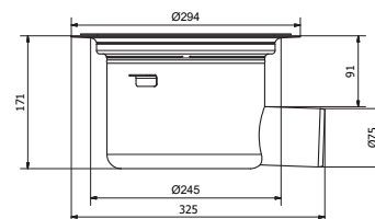
Sida Ø75 mm (Syrafast rostfritt stål)
